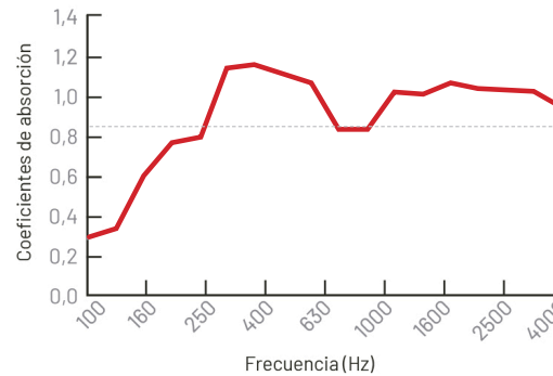
Gráfico de absorción de sonido en base a su frecuencia.
