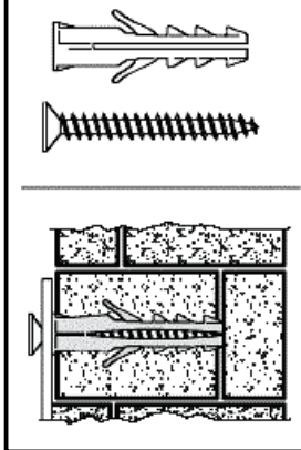
"FISCHER" Nylon plug
