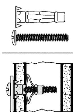
TASSELLO METALLICO AD ESPANSIONE
