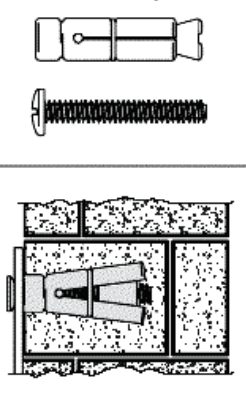
TASSELLO DI ANCORAGGIO IN METALLO
