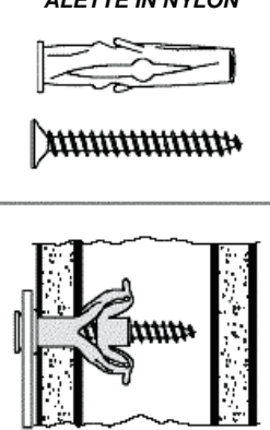
TASSELLO DI ANCORAGGIO AD ALETTE IN NYLON
